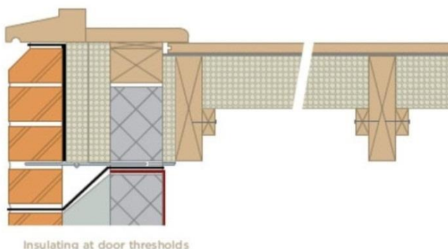
Izolația la pragul ușii
