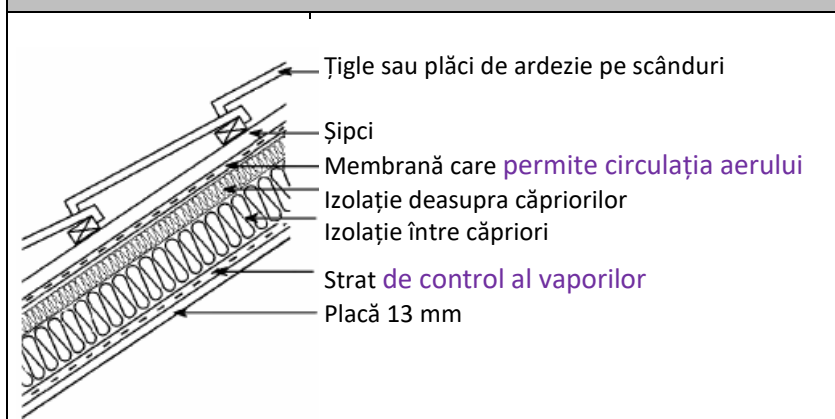
Diagrama B4: Izolație deasupra și între căpriori
