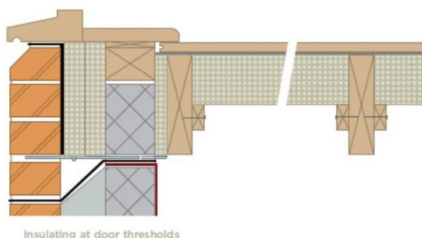
Izolația la pragul ușii
