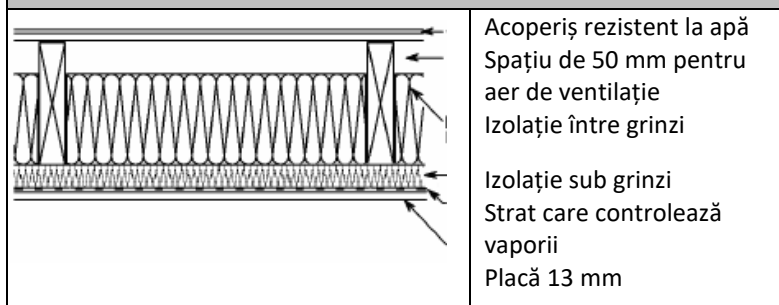
Diagrama B5 Acoperiș plat din lemn, izolație între și sub grinzi
